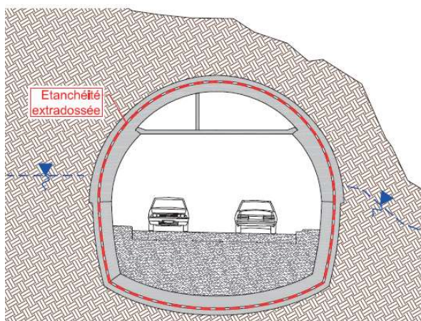
FIGURES 1 – Exemples de schémas de principe de tunnel creusé
