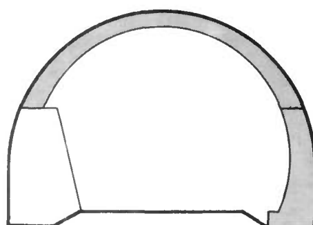
Realisation des piedroits par plots alternés
