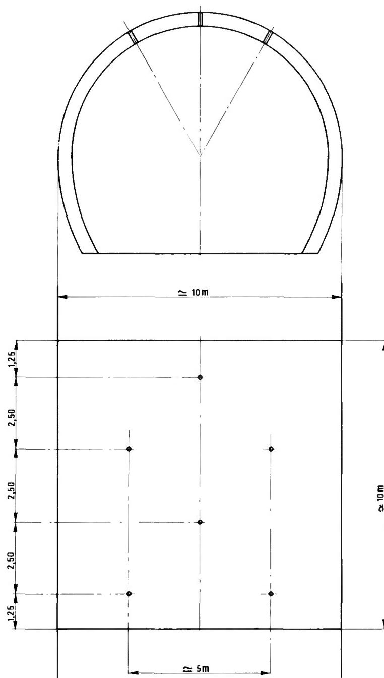
Figure 35. Schéma type de la répartition des forages pour injection de remplissage.
