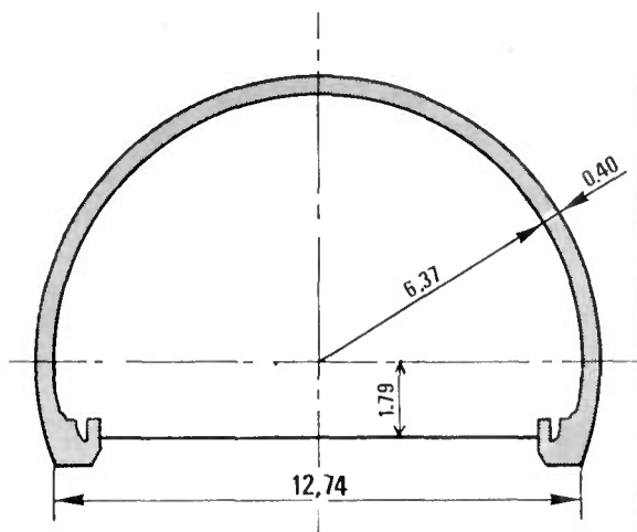
Autoroute A 8 Tunnels à 3 voies de circulation
