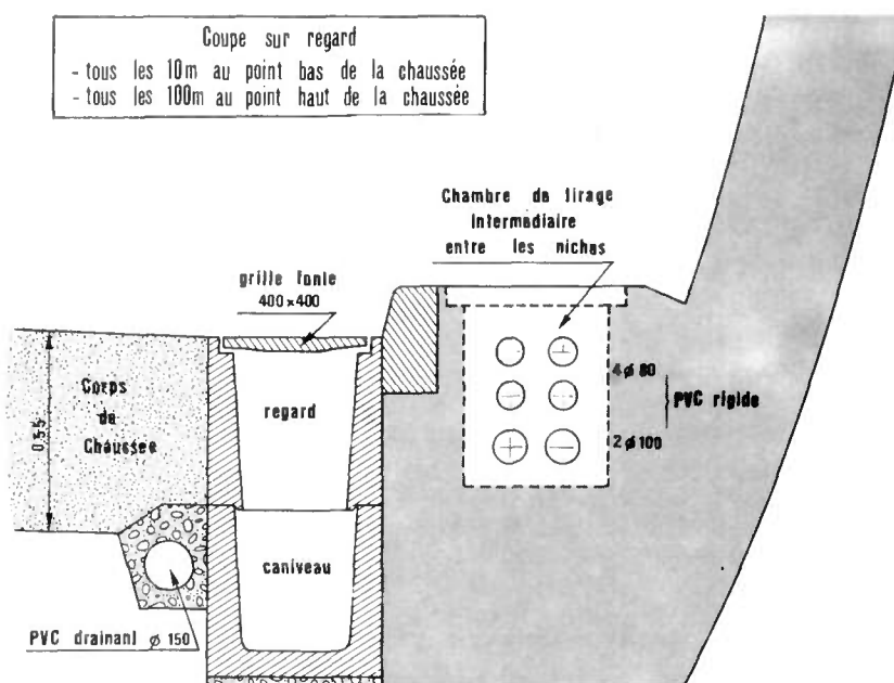
Figure n  4. Autoroute A 40 -Tunnel de Chamoise. Am nagement type des banquettes
