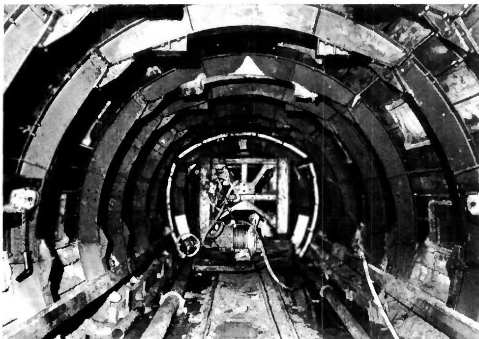
Figure 20. Galerie technique sous Fourvière - Lyon. Élément de coffrage en cours de transfert sous un autre élément en position coffrante.
